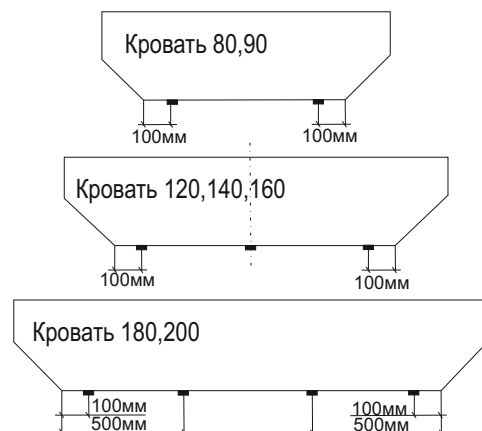
Схема установки подпятников
